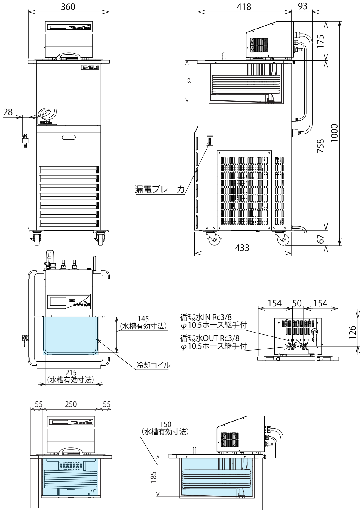
■ 水槽部 槽内有効寸法: 215W×145D×150Hmm
